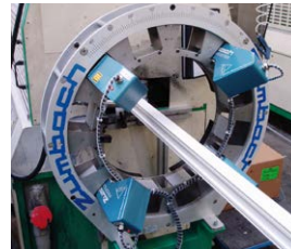
PMM 140D-4A Mesure des profilés de portes et de fenêtres.
